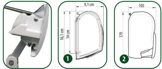
Markise, 3 Wandhalterungen inklusive Befestigungsmaterial mit Abdeckklappen und teleskopierbarer Kurbel.
