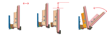
Tiefe 20 mm Höhe 39 mm Neigungswinkel -10° / +45°
